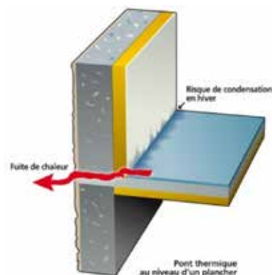
Schéma de principe des ponts thermiques à la liaison plancher intermédiaire / voile de façade
